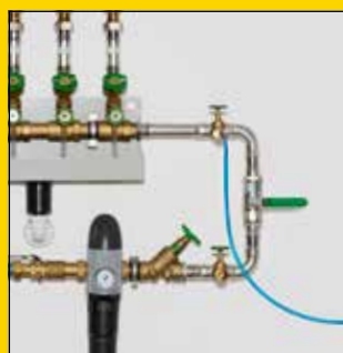
Tlačni preizkus z stisnjenim zrakom (SL/SWL)
