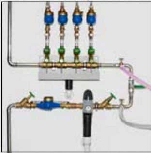
Izpiranje napeljav za pitno vodo (S/SL/SLW)
